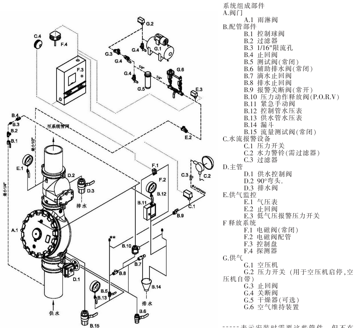
电启动单连锁预作用阀组系统图
