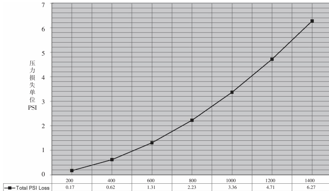
DN100 止回阀 流量-压力损失曲线 流量单位:加仑/分(GPM)
