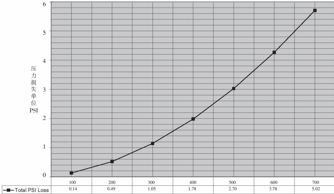
DN150 止回阀 流量-压力损失曲线 流量单位:加仑/分(GPM)
