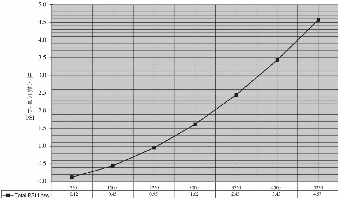
DN200 止回阀 流量-压力损失曲线 流量单位:加仑/分(GPM)
