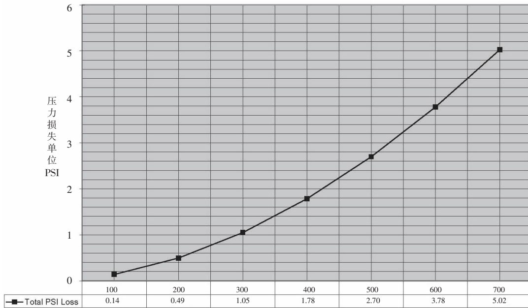
DN80 止回阀 流量-压力损失曲线 流量单位:加仑/分(GPM)
